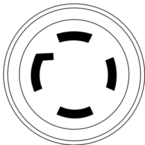
Figura 2-6. Tomacorriente de 120/240 VCA, 30 A NEMA L14-30R
