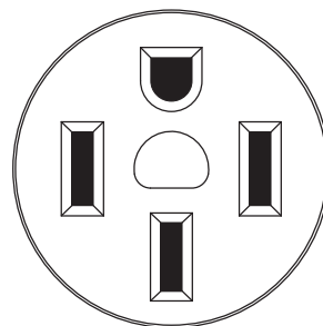
Figura 2-7. Tomacorriente de 120/240 VCA, 50 A NEMA 14-50
