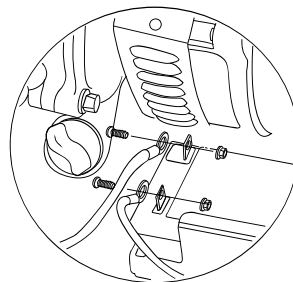
Figure 4-5. Conexión de la batería
