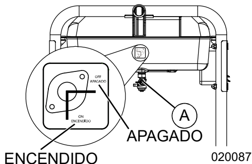
Figura 3-2. Válvula de corte del combustible
