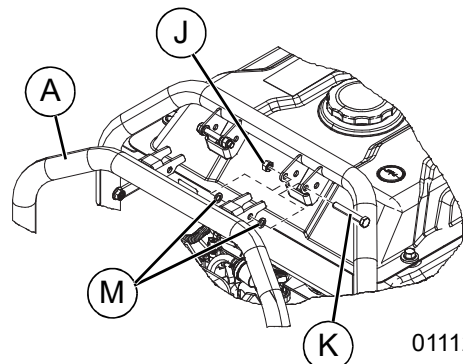
Figura 2-10. Ensamblaje de la manija
