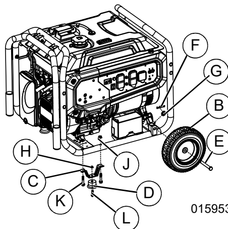
Figura 2-9. Ensamblaje de la rueda y la pata
