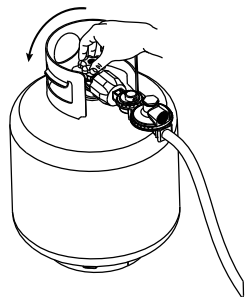
Figura 2-16. Abra la válvula de tanque de PL
