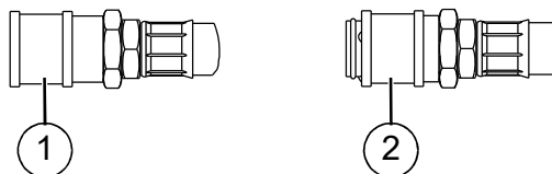
Figura 2-19. Manguito deslizable
