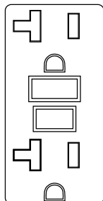
Figura 2-5. Tomacorriente doble de interruptor de circuito por falla de conexión a tierra (GFCI) de 120 VCA, 20 A (NEMA 5-20R)
