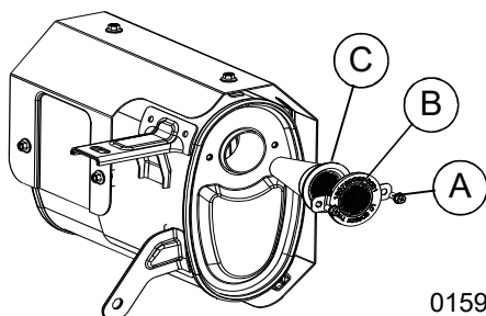
Figure 4-6. Pantalla del supresor de chispas
