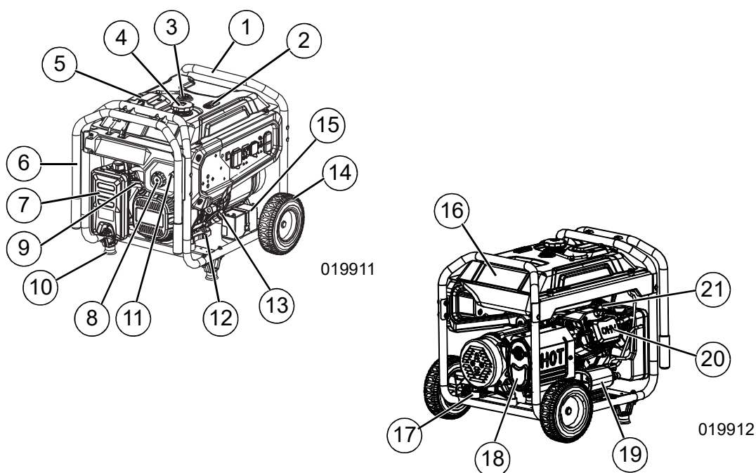
Figura 2-1. Características y controles
