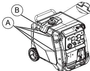
Figure 4-3. Porte d'accès
